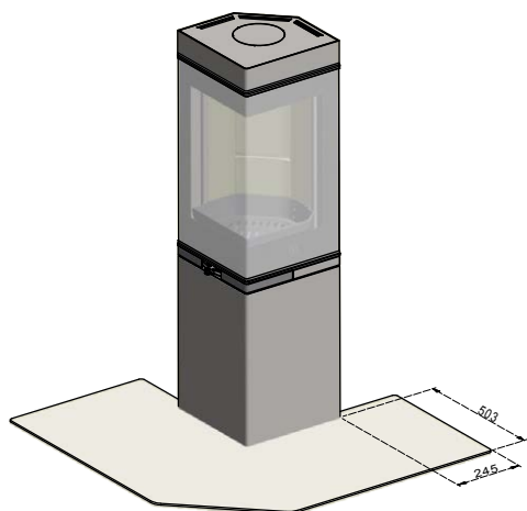
Pedana grande in vetro trasparente o grigia fumo per la serie Scan 80
