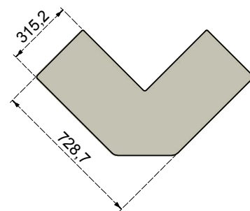
Pedana piccola ad angolo in vetro trasparente fumo
