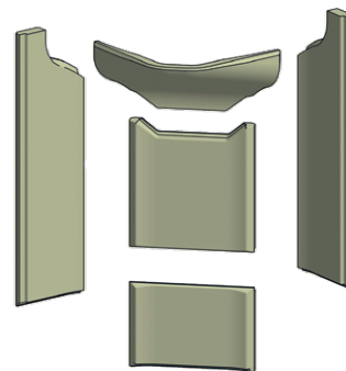
Rivestimento della camera di combustione
