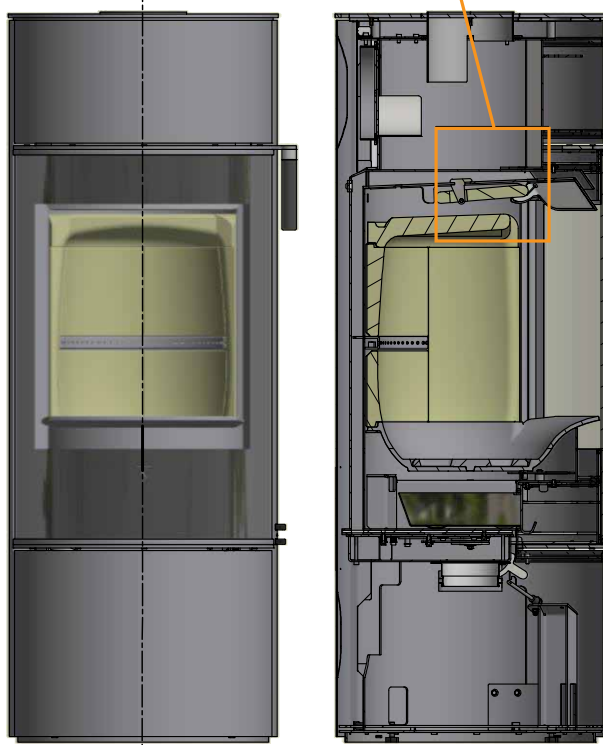
Piastra deflettore fumi superiore
