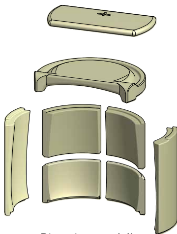
Rivestimento della camera di combustione
