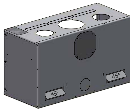
Cassetta senza piastre di copertura per connettori di convezione
