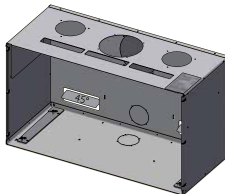
Cassetta senza piastre di copertura per la convezione dell'aria
